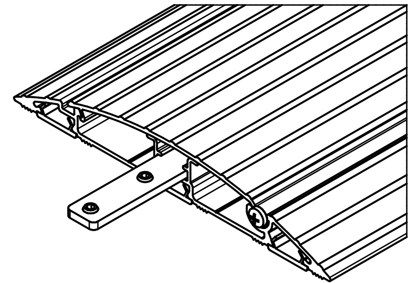
standaard connection strip schroefjes van boven bereikbaar
