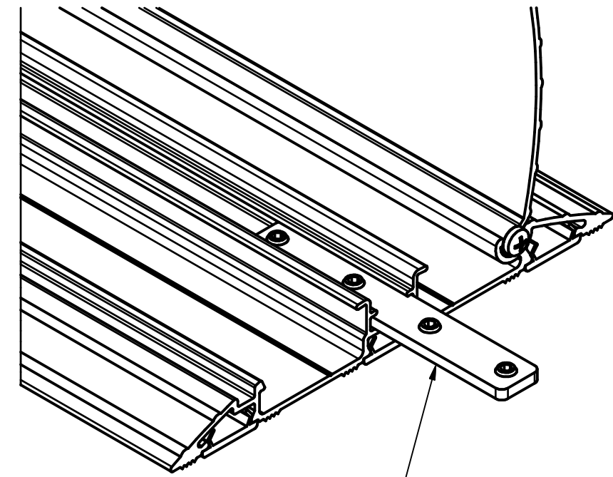
standaard connection strip schroefjes van boven bereikbaar
